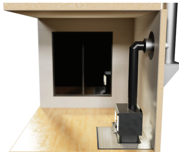
INSTALLATION TRAVERSANT UN MUR
